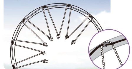
バスケットネット取付例(下から見た図)
